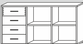
00063L/40/F/G* 134x70x40cm (BxHxT) 00063L/32/F/G* 134x70x32cm (BxHxT)
