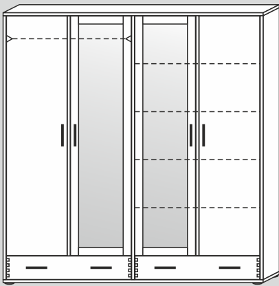
00020/F/G* 178x182x56cm (BxHxT)
