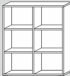
00047/40/F* 90x102x40cm (BxHxT) 00047/32/F* 90x102x32cm (BxHxT)
