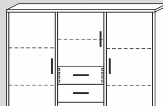
00017L/40/F/G* 134x102x40cm (BxHxT) 00017L/32/F/G* 134x102x32cm (BxHxT)
