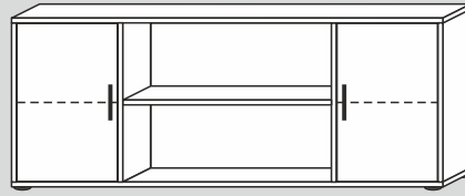
00077/40/F/G* 178x70x40cm (BxHxT) 00077/32/F/G* 178x70x32cm (BxHxT)
