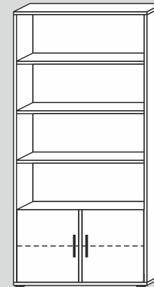
00040/40/F/G* 90x182x40cm (BxHxT) 00040/32/F/G* 90x182x32cm (BxHxT)
