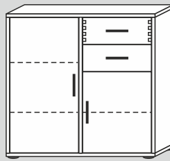
00037L/40/F/G* 90x86x40cm (BxHxT) 00037L/32/F/G* 90x86x32cm (BxHxT)
