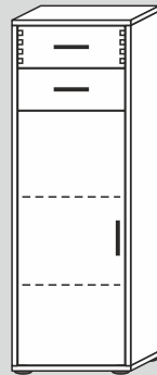
00010L/40/F/G* 46x134x40cm (BxHxT) 00010L/32/F/G* 46x134x32cm (BxHxT)
