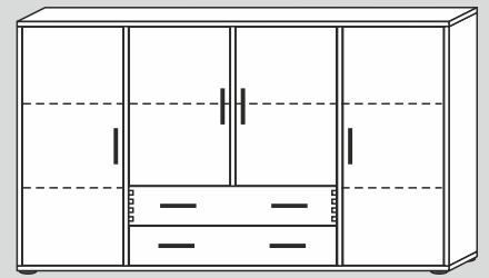
00014/40/F/G* 178x102x40cm (BxHxT) 00014/32/F/G* 178x102x32cm (BxHxT)
